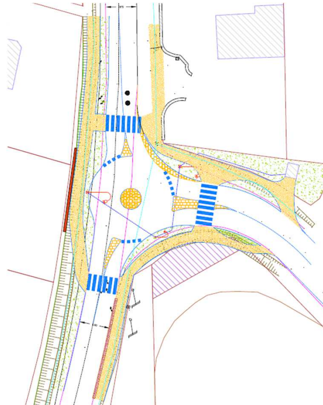
Aménagement de sécurité - giratoire de Trélivalaire
