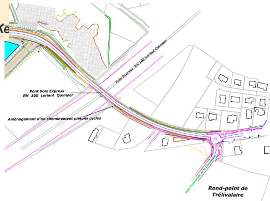
Aménagement de sécurité entre giratoire de Trélivalaire et impasse de Trélivalaire
