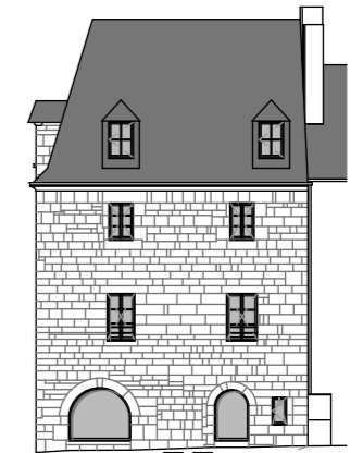
FACADE NORD PROJET sur rue Isolé
