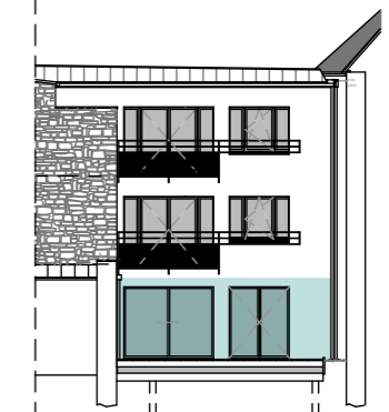
FACADE OUEST SUR JARDINET
